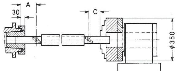
Spannfutter
