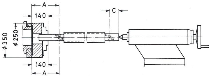
Dreibackenfutter
